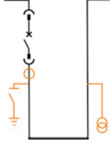
Vakum Kesicili Kuplaj ve Bara Yükseltme Panosu
