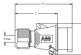
Ölçüler (mm)
