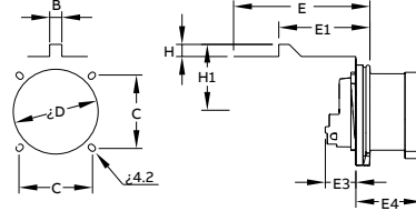
Ölçüler (mm)
