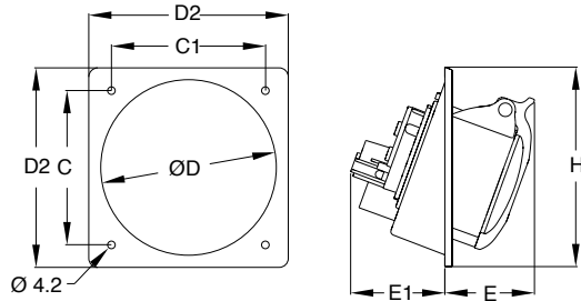
Ölçüler (mm)
