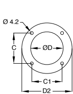
Ölçüler (mm)
