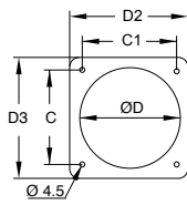
Ölçüler (mm)
