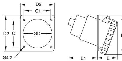
Ölçüler (mm)
