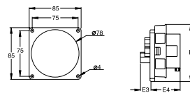
Ölçüler (mm)
