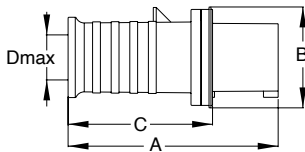
Ölçüler (mm)
