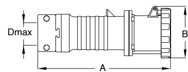
Ölçüler (mm)
