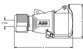
Ölçüler (mm)
