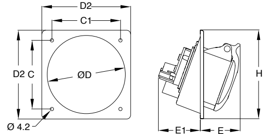
Ölçüler (mm)
