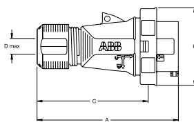
Ölçüler (mm)
