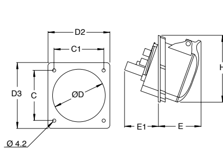
Ölçüler (mm)
