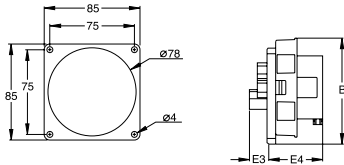
Ölçüler (mm)
