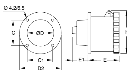
Ölçüler (mm)
