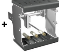
Sabit şalteri çekmeceli tipe dönüştürme kiti
