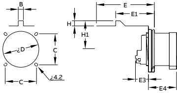
Ölçüler (mm)
