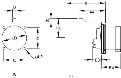
Ölçüler (mm)
