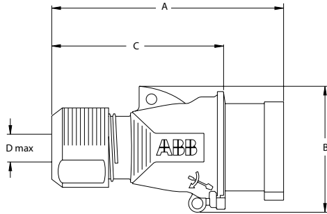
Ölçüler (mm)
