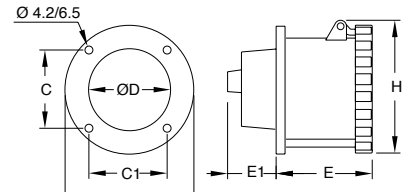
Ölçüler (mm)
