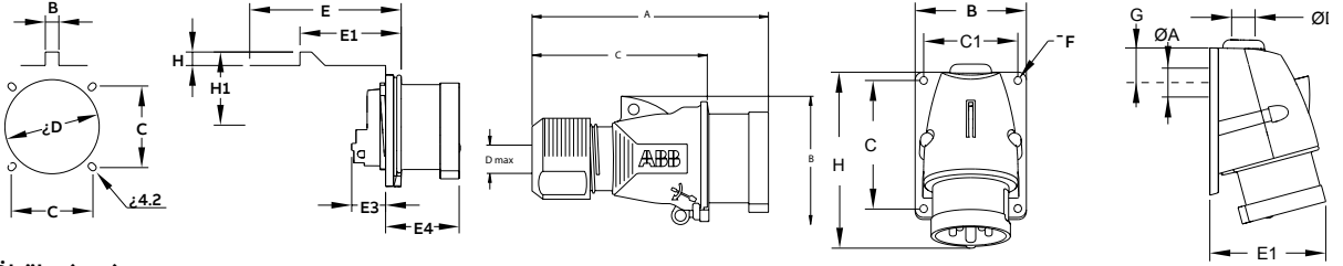
Ölçüler (mm)
