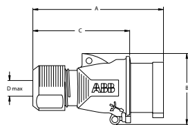
Ölçüler (mm)
