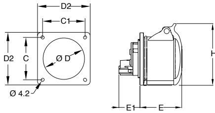
Ölçüler (mm)
