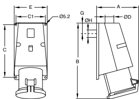
Ölçüler (mm)
