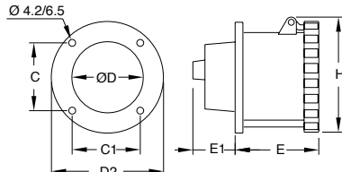
Ölçüler (mm)
