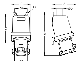
Ölçüler (mm)
